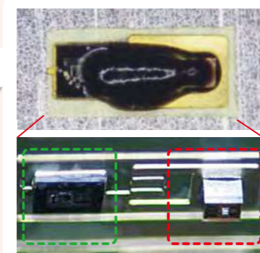
試作機の左側が0.6ミリメートル角のグルコース発電素子、右側が約0.4ミリメートル角の送信回路。グルコース発電素子が電力源とセンシングを行い、送信回路がグルコース濃度を無線送信頻度に変換、送信する。
