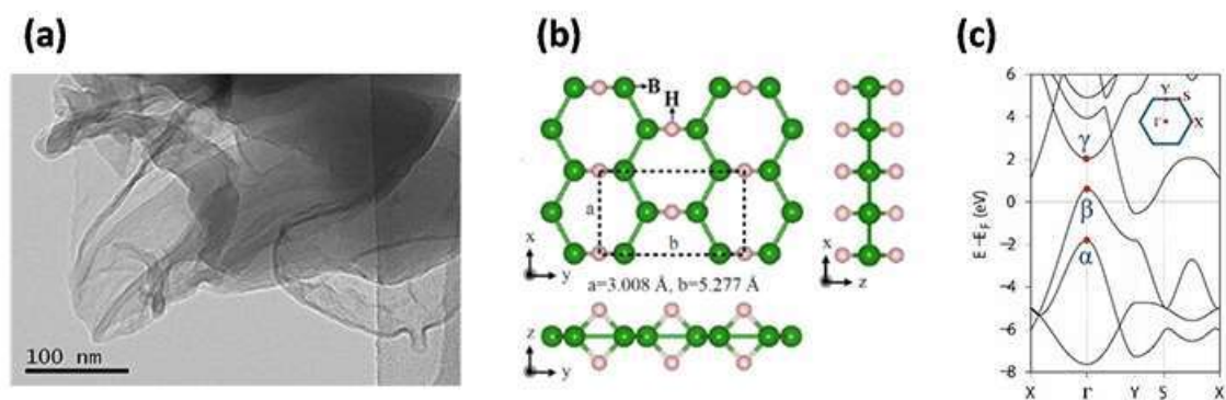
図2. ホウ化水素シートの透過型電子顕微鏡写真 (a)、結晶構造 (b)、電子構造 (c)
