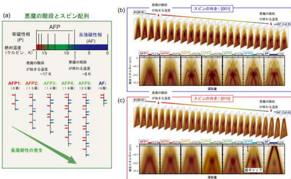
図2： (a) 「悪魔の階段」に対応する長周期スピン配列の変化。(b)(c) 磁気ドメインを選択したレーザー光電子分光で観測した「悪魔の階段」に伴う電子構造の変化。電子構造と共に、(c)では擬ギャップの温度変化も観測されました。この結果は、「悪魔の階段」を発生させる長周期のスピン配列が伝導電子の擬ギャップ状態に由来していることを意味しています。
