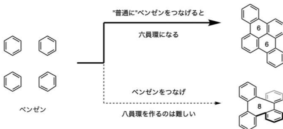
図2 従来の環構造を構築する手法
