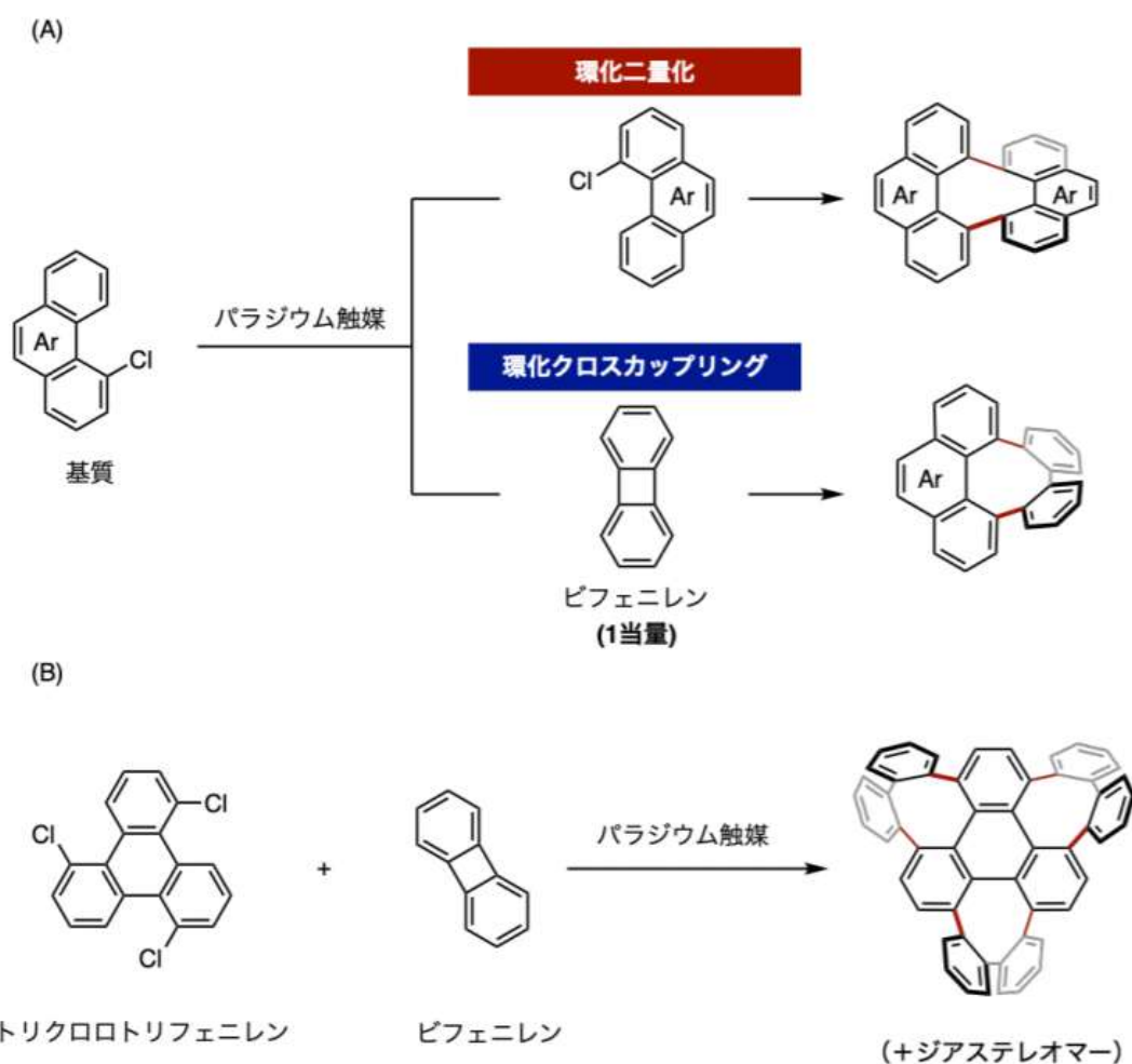
図3 本研究で達成した合成反応
