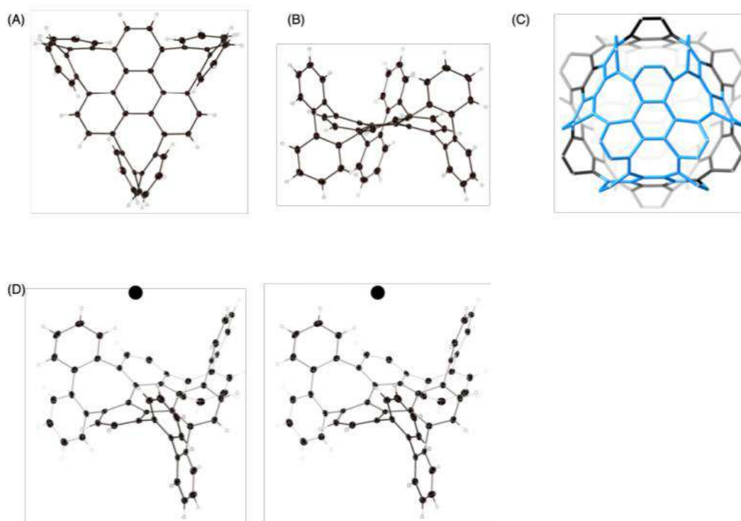
図4 三連続八員環構築反応で合成した分子
