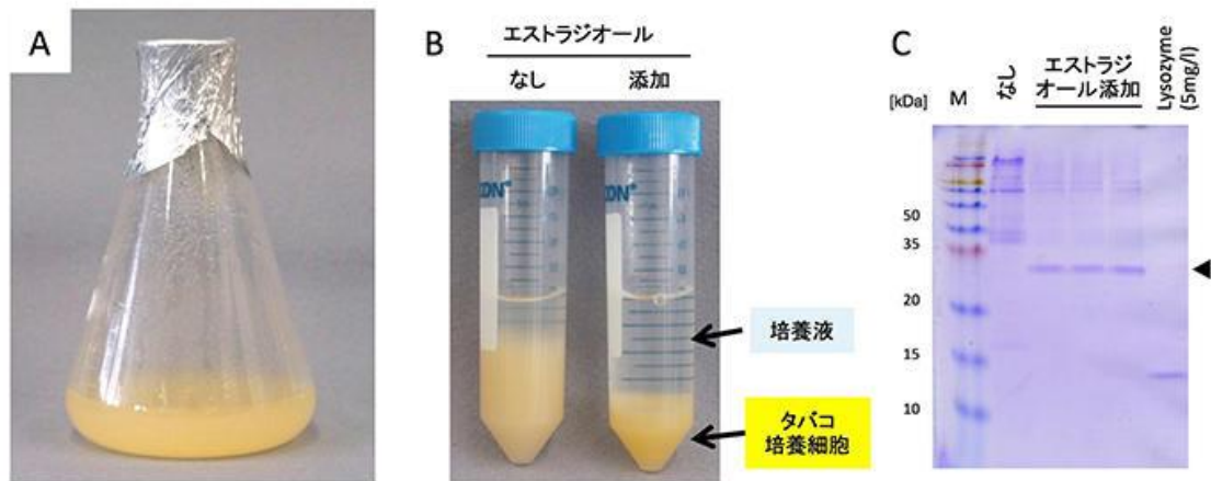
図2: タバコ培養細胞を用いた ORF8 タンパク質の合成
