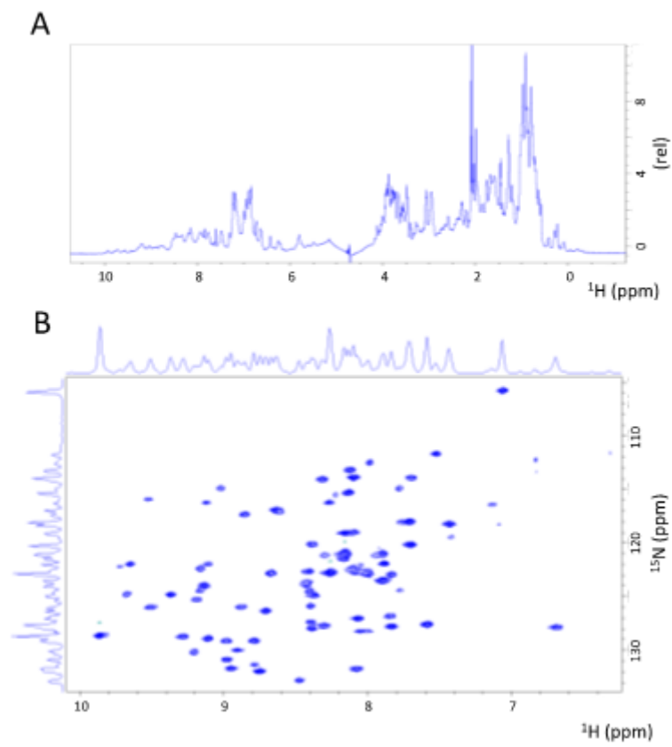
図3: ORF8 タンパク質の NMR スペクトル
